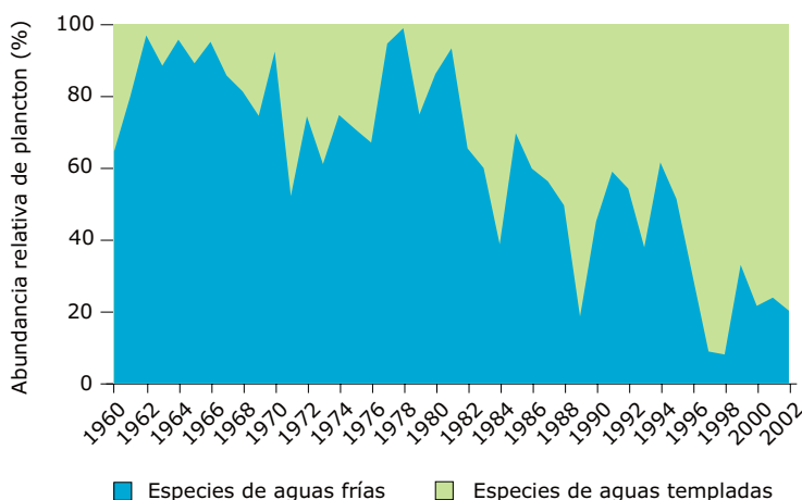
Datos sobre dos especies de copépodo encontradas en el Mar del Norte central aguas templadas: Calanus helgolandicus y aguas frías: Calanus finmarchicus
