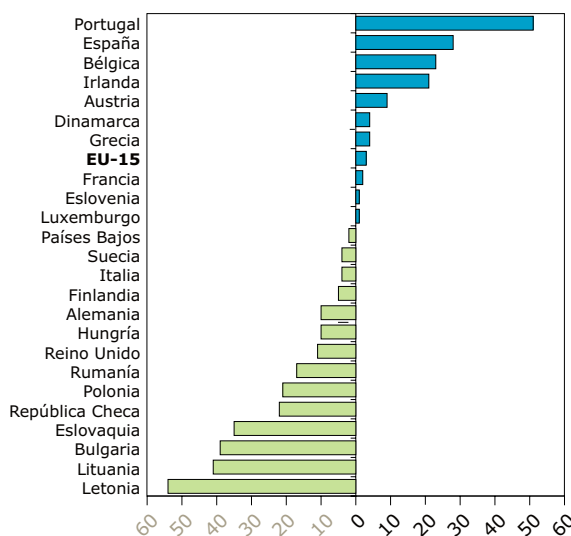
Diferencia entre las emisiones de precursores* del ozono y la Directiva sobre Límites de Emisiones Nacionales, o los objetivos del Protocolo de Gotemburgo (Distancia en puntos porcentuales entre las emisiones observadas en el 2001 y las emisiones (teórico-lineales) en el 2001 necesarias para el cumplimiento de los objetivos)
